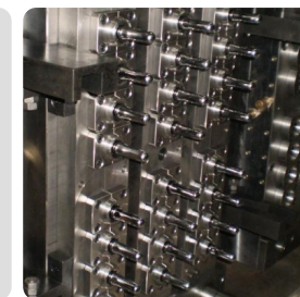
热流道模具 Hot runner mold
