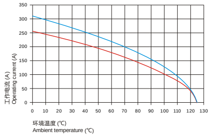
D2MK-001-F(25-40mm 2 ) D2MK-001-F(40-70mm 2 )
